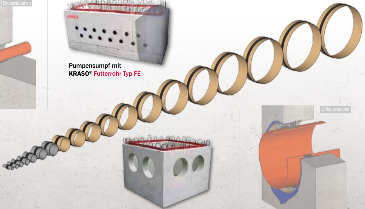
Pumpensumpf mit KRASO® Futterrohr Typ FE/MI
