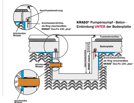
Bauquerschnitt
