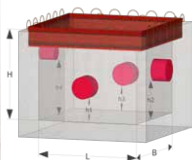
Anordnung der Anschlüsse bei Standardgrößen
