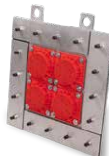
KRASO® Kabeldurchführung KDS 150 FL/ZA als Mehrfachdichtpackung - mit Fest- Losflansch und Vorbauflansch FDS 150 auf der Außenseite, Zum Andübeln (Sonderanfertigung)
