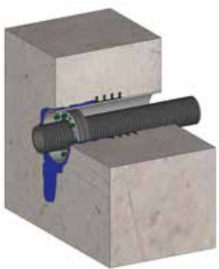
Einbausituation mit KRASO® Dichteinsatz Typ GR
