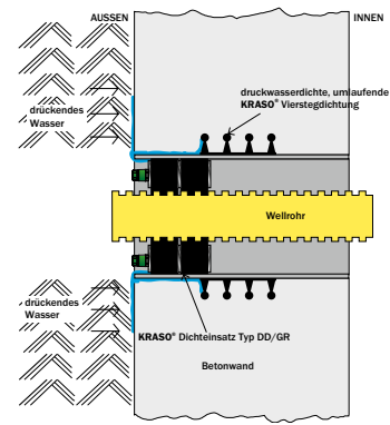
Bauquerschnitt
