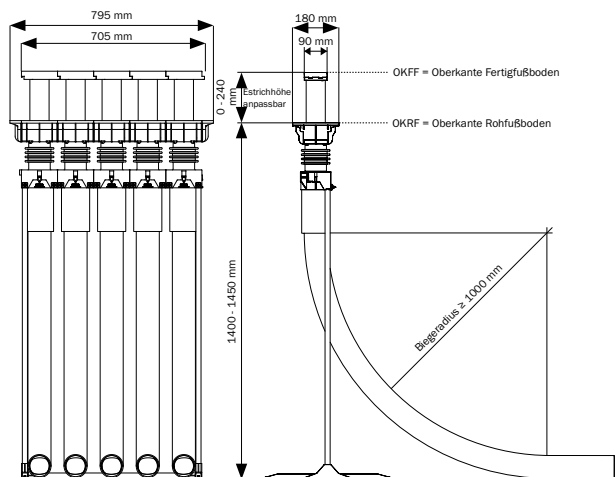
Technische Zeichnung - 5-fach
