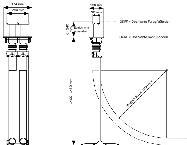
Technische Zeichnung - 2-fach
