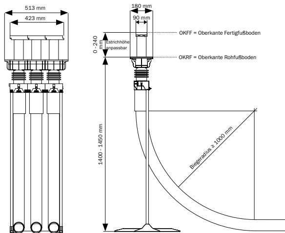
Technische Zeichnung - 3-fach
