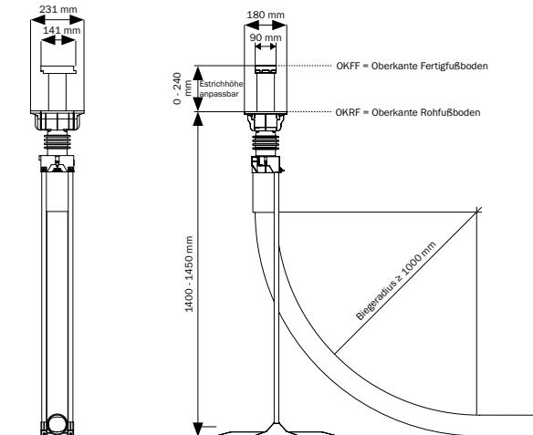
Technische Zeichnung - 1-fach
