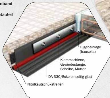
KRASOflex® Klemmkonstruktion - außenliegend
