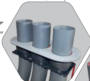
KRASO® KDS 150 opzetstuk voor mantelbuis Voorbeelden van leidingdoorvoeren met KRASO® klemdichtringen
